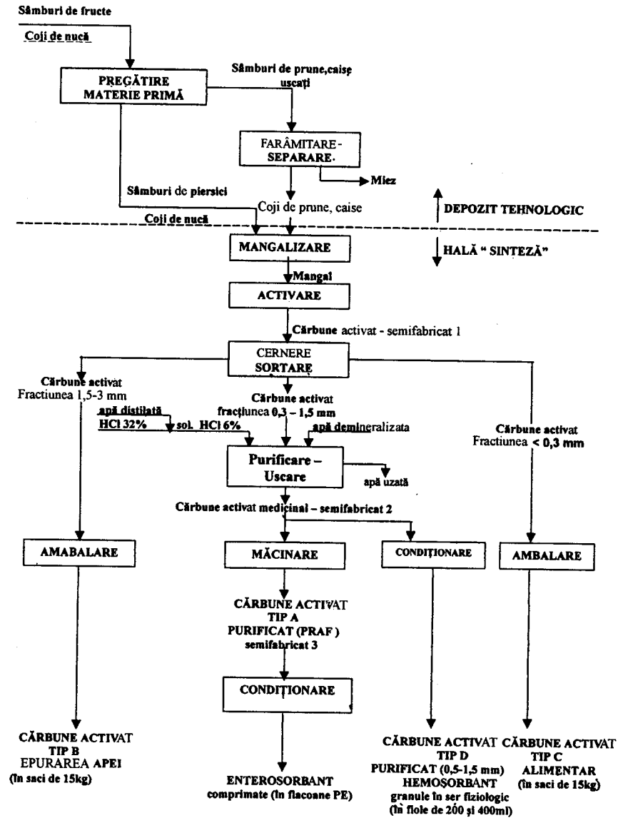
Schema fluxului tehnologic al procedurii de obținere a cărbunelui activat din sămburi de fructe și coji de nucă
